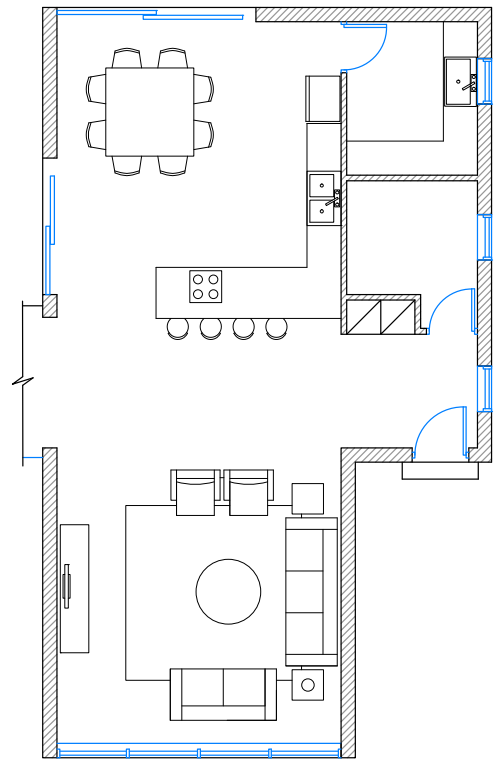
ΚΑΤΟΨΗ ΚΛΙΜΑΚΑ 1:100
